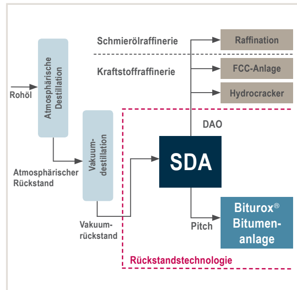
Abb. 2: SDA-Anlage als Bestandteil einer modernen Rückstandstechnologie
